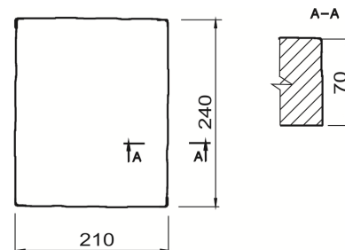
Krycia platňa:
