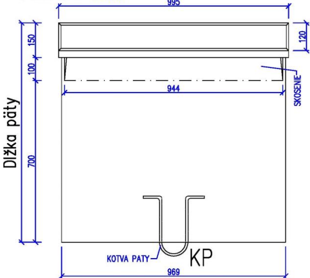
PODORYS M=1:10
